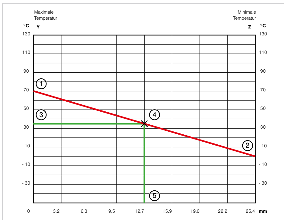
Rys. 3: Przykład ustalania odstępu kompensacyjnego
