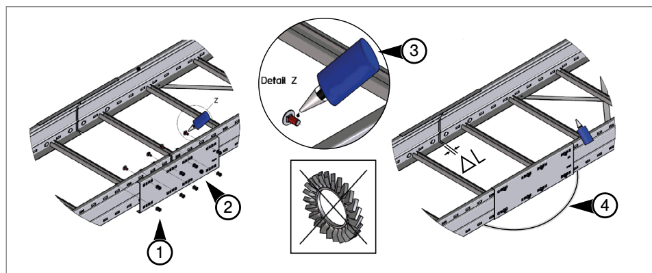
Rys. 4: Montaż łączników jako podpory przesuwnie
