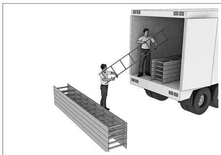
Rys. 1: Rozładunek tras kablowych
